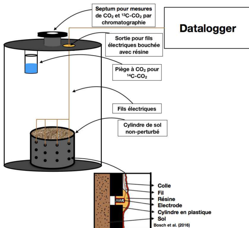
Figure 1 : Dispositif expérimental microcosme (partie principale) contenant échantillon de sol non-perturbé équipé d'électrodes. Les microcosmes ont un piège à CO 2 pour les analyses de 14 C et un septum pour les prélèvements de gaz pour les analyses de CO 2 et 13 C-CO 2 . Les mesures de 14 C et 13 C seront faites en parallèle sur des microcosmes identiques.
